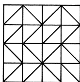
Fig. 6a. \Omega = (0,1)^2 , n = 2
